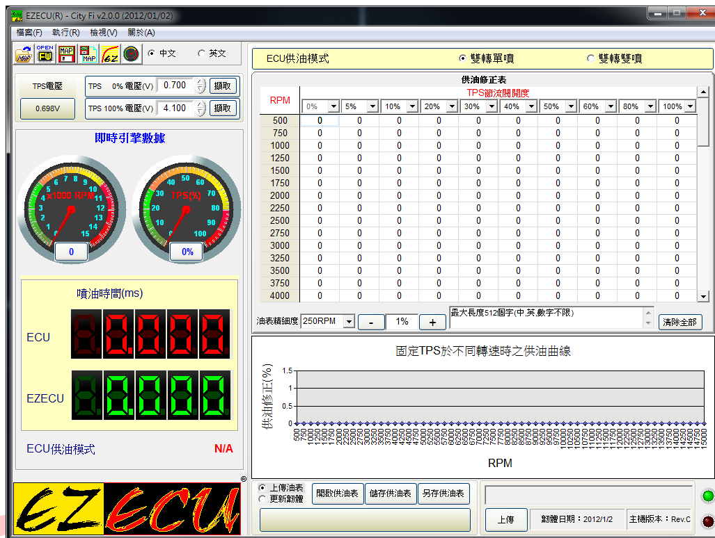
圖 3-2 City Fi ECU 應用軟體操作畫面 (已連線)
